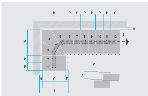
vista in pianta con ingombri
