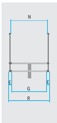
vista frontale con 2 lati di ringhiera
